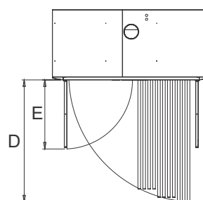
TS-93 TOP
